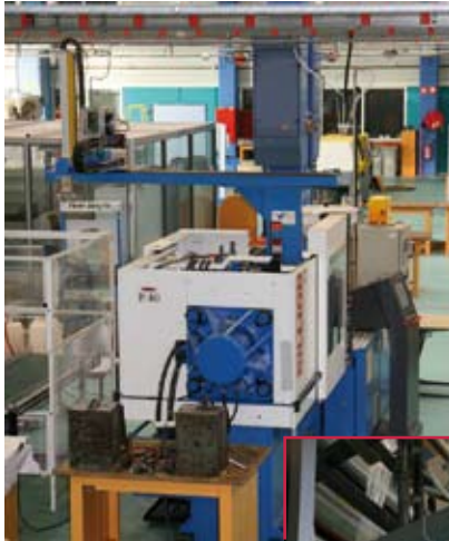
Presse d'injection équipée d'un robot
